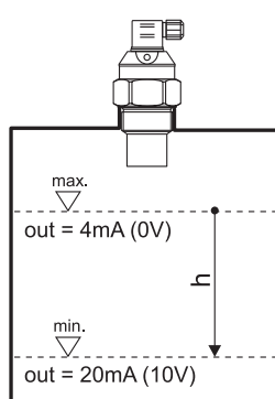
Fig 34: Modo inverso
