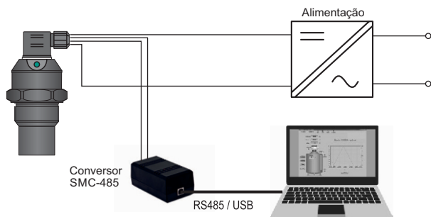
Fig 35: Configuração padrão do hardware com Modbus®
