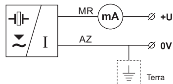
Conexão elétrica para saída de corrente (opção C)
