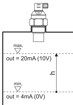
Fig 33: Modo padrão
