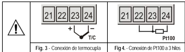
Fig. 3 - Conexión de termocupla
