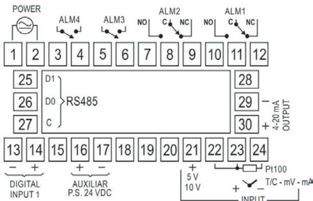
Fig. 1 - Conexiones del panel trasero
