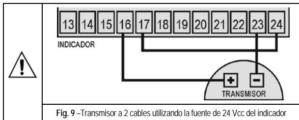
Fig. 9 –Transmisor a 2 cables utilizando la fuente de 24 Vcc del indicador
