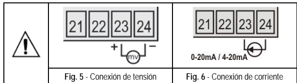
Fig. 5 - Conexión de tensión
