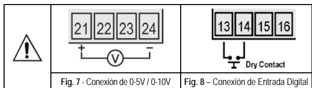
Fig. 7 - Conexión de 0-5V / 0-10V
