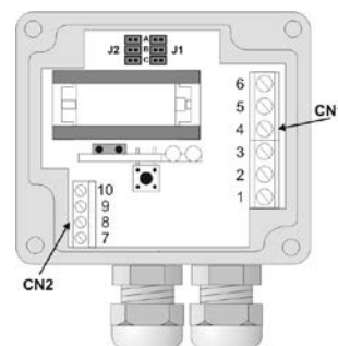
Fig. 8 – Versión IP65, vista interna de las conexiones
