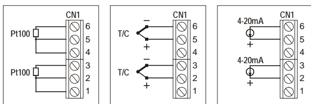
Fig. 10 – Conexiones del señal de entrada
