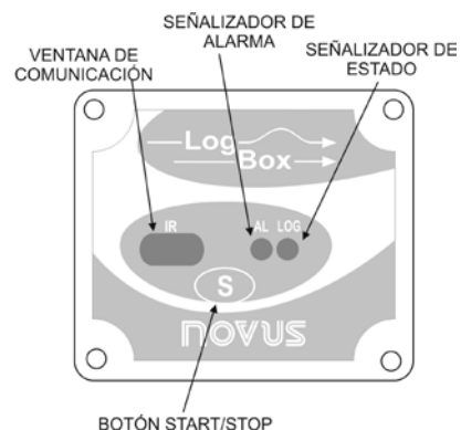
Fig. 2 – Señaladores y ventana de comunicación IR
